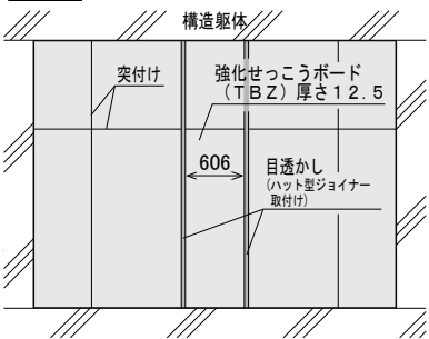
正面図
