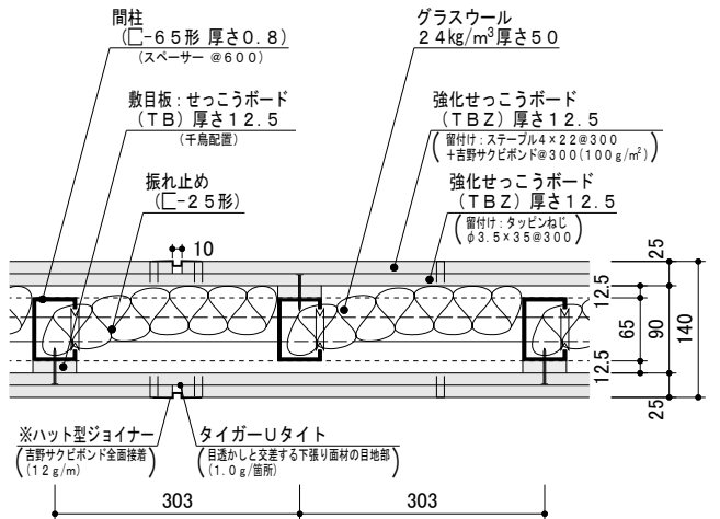
水平断面図
